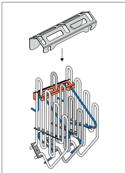
3. attēls HUUM DROP 4 un 6 atdalītājrežģa uzstādīšana ar 3 sildelementiem.
